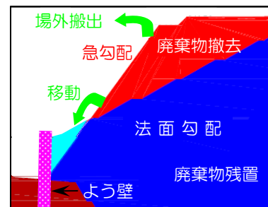
< 整形工事概略図 >
