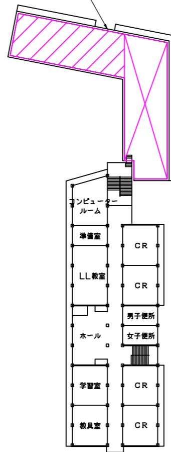
4階平面図
