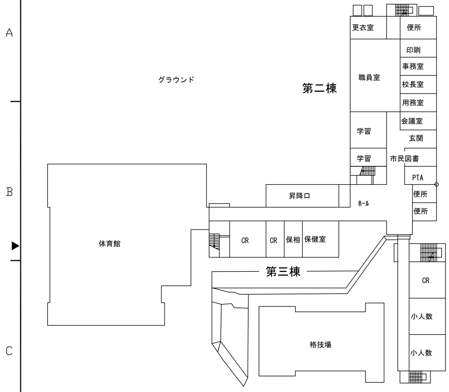
配置図・1階平面図（第一棟：2階）
