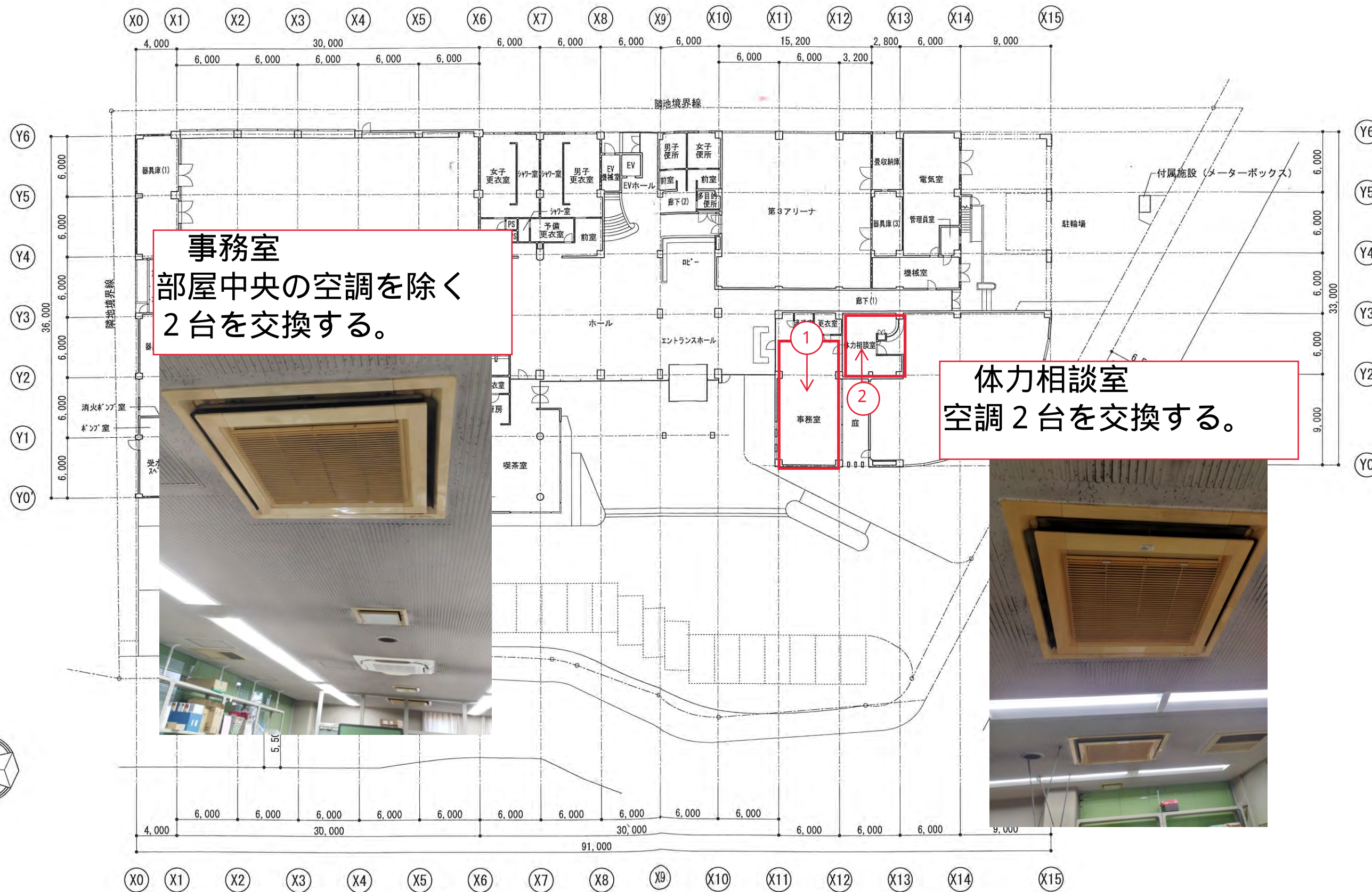
配置図兼 1階平面図 S=1/400
