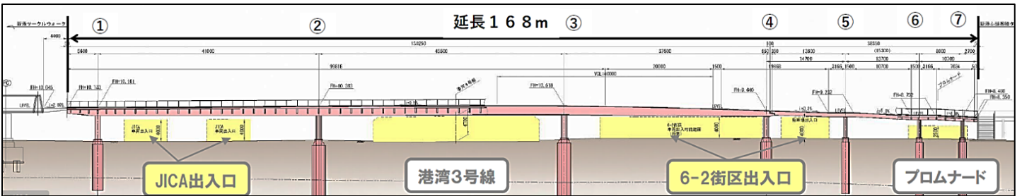
【立面図】
