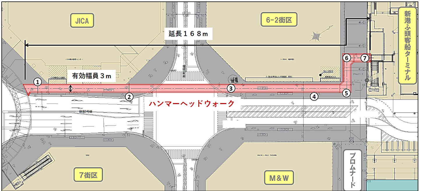
【配置図】
