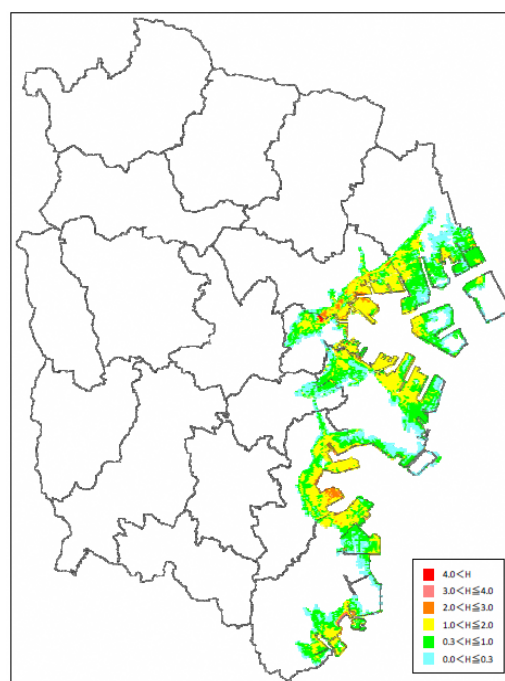
[慶長型地震]
