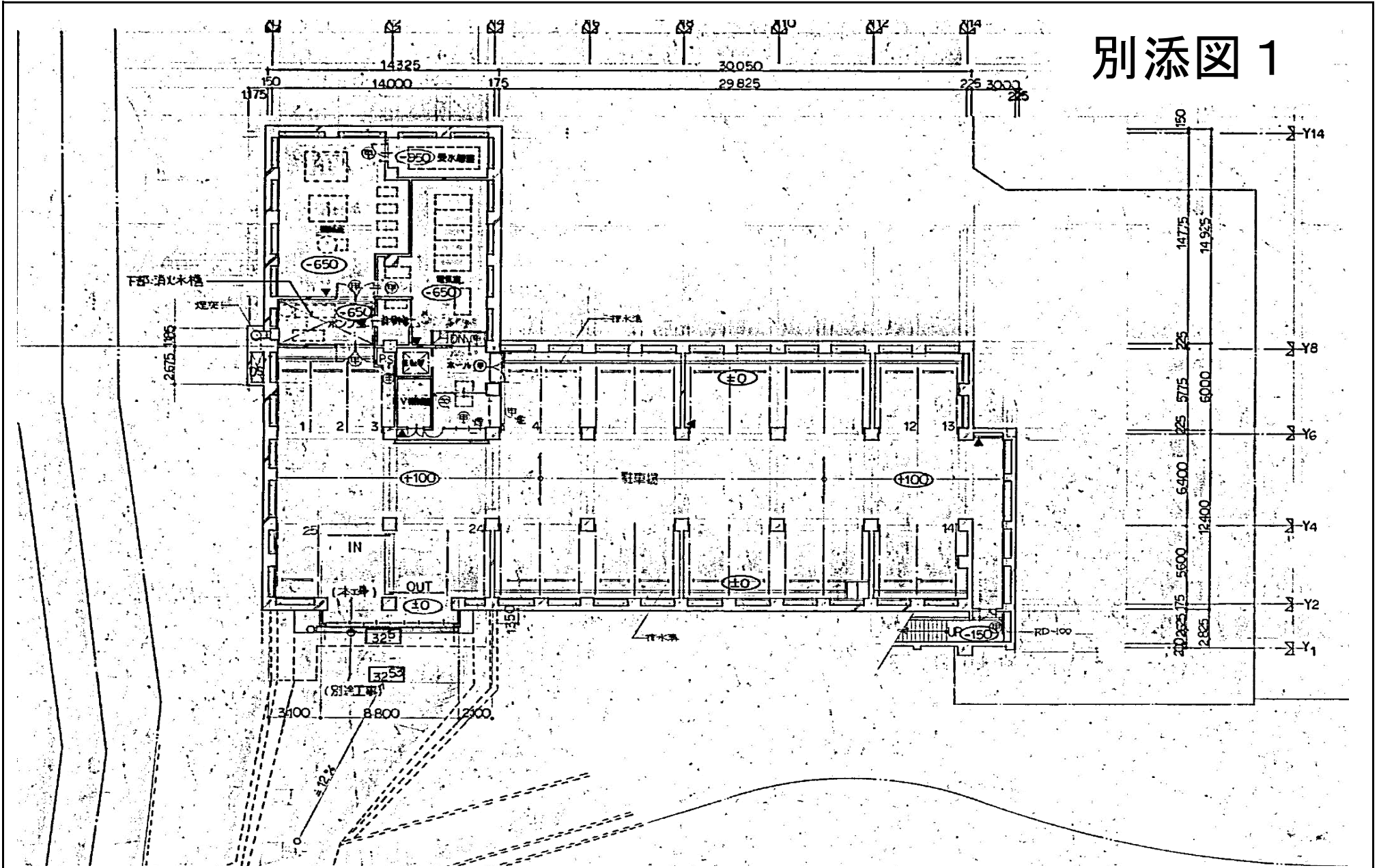
図名 神奈川スポーツセンター平面図 (地下1階)
