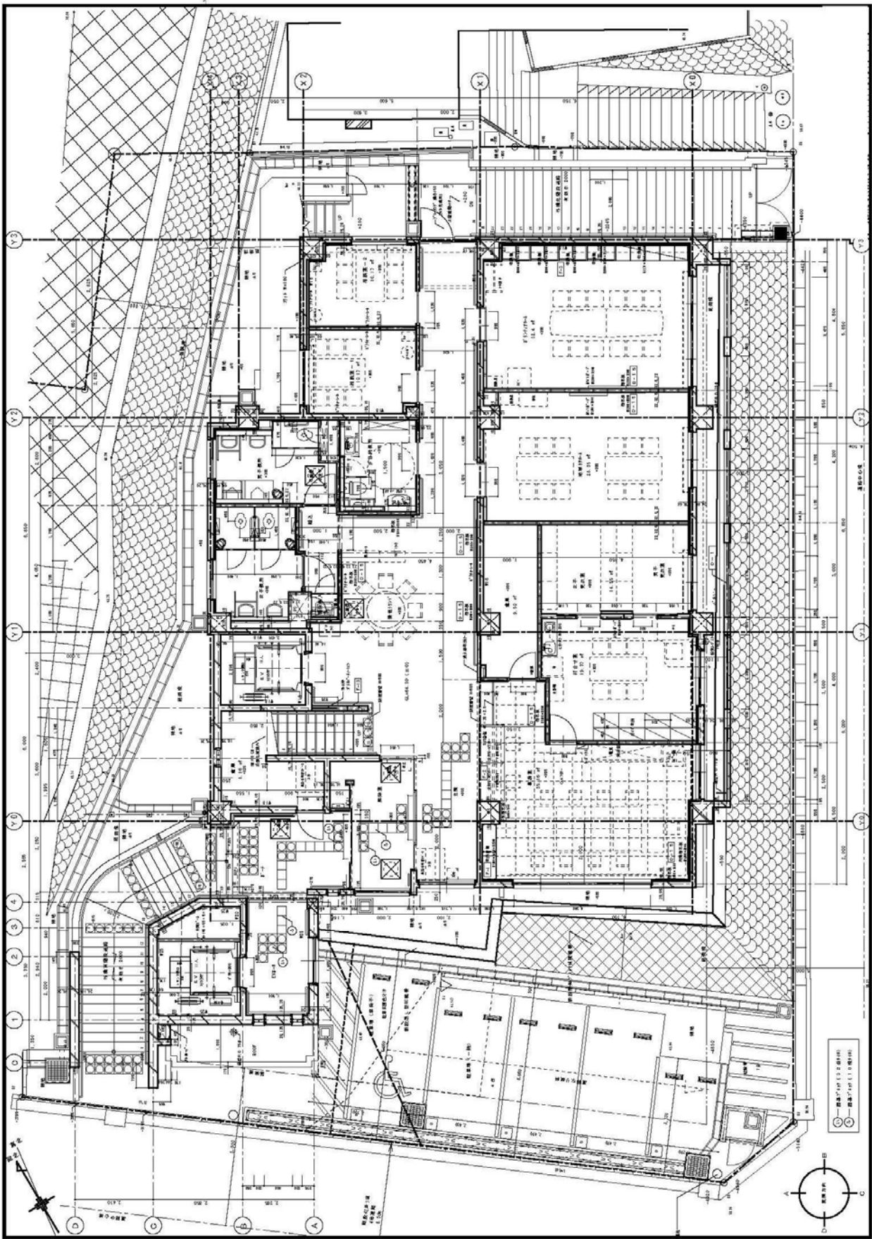
<1 階平面図>
