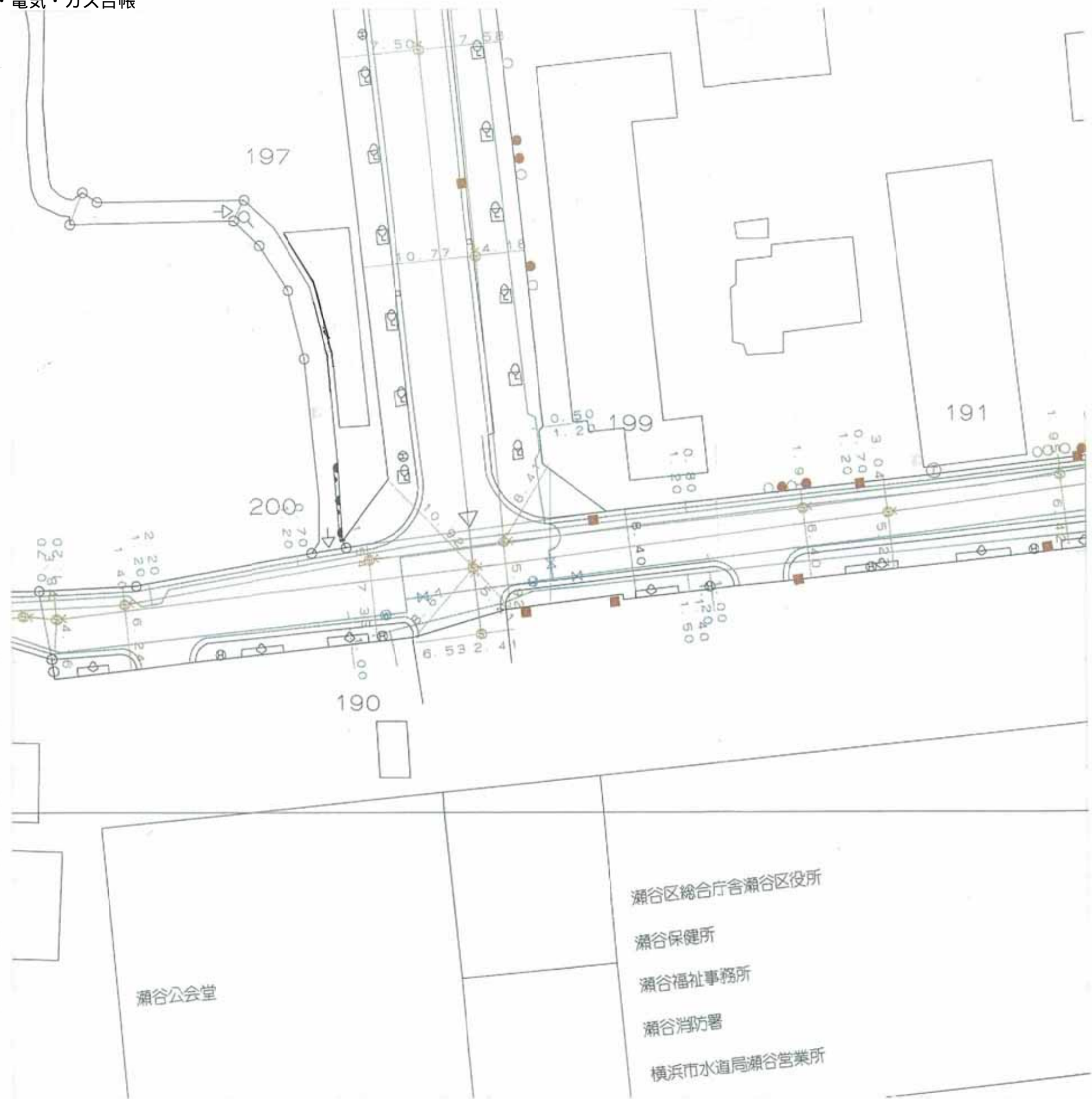
図面番号: 201237
