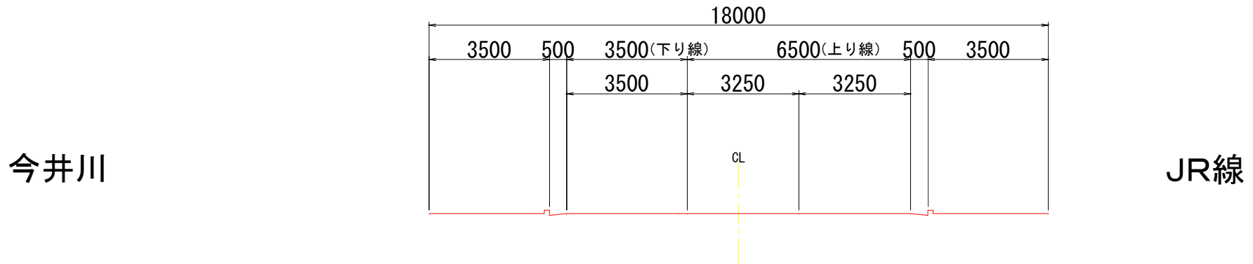
現況横断図
