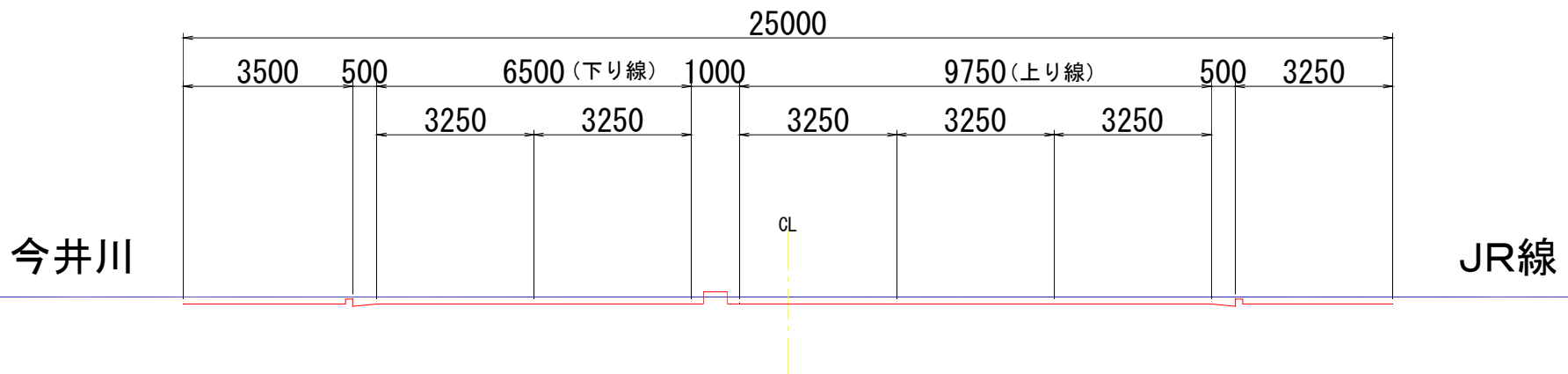
計画横断図
