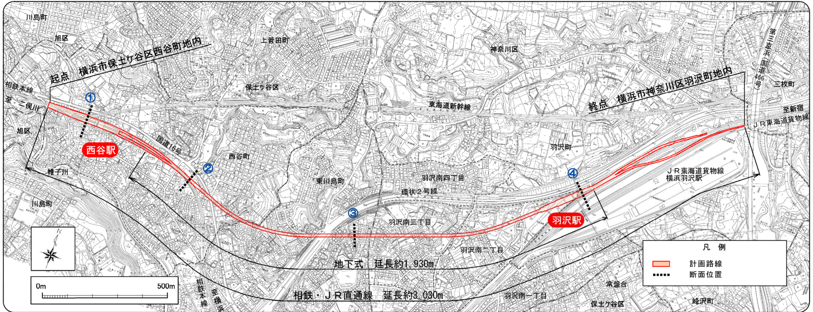
図 1-1(1) 平面図
