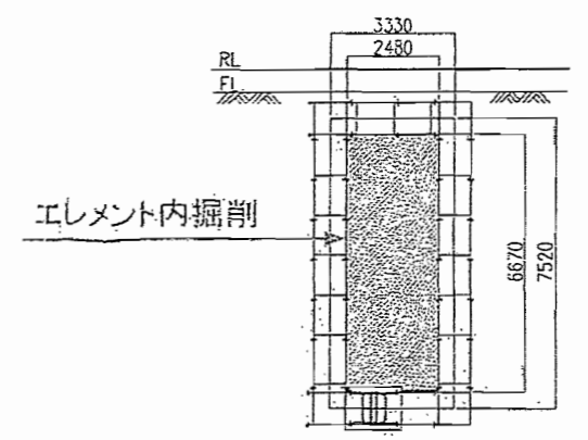
A-A断面図 S=1/200 仮水路2
