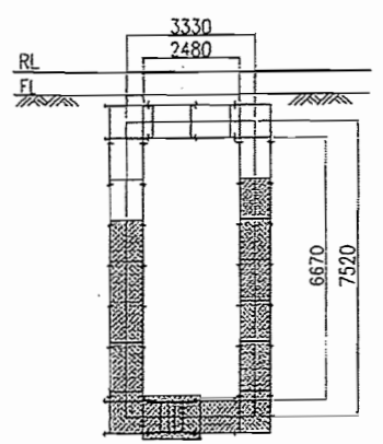
A-A断面図 仮水路2 S=1/200
