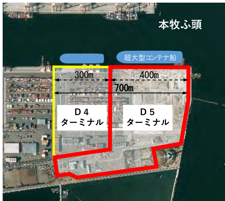
D5ターミナル平面図
